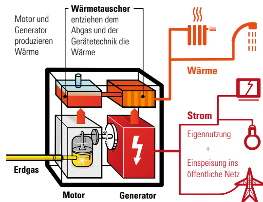
Darstellung Funktionsweise Mini-BHKW individuell
